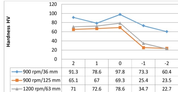
شکل 7- پروفیل سختی نمونه‌های جوشکاری شده.
