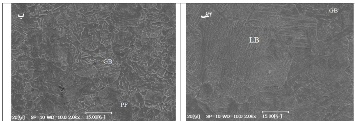
شکل ۴- تصویر میکروسکوپی الکترونی روبشی از ناحیه جوش در سرعت پیشروی 20 mm/min در دو موقعیت متفاوت SZ ؛ الف: مرکز SZ ؛ ب: SZ در نواحی نزدیک به HAZ.
