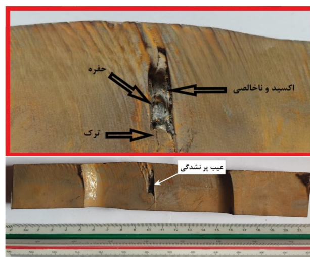
شکل 18- نمای مقطع عرضی نمونه جوشکاری شده پس از وایرکات، که ناحیه دارای عیب پرنشده کامل در ریشه جوش را نشان می‌دهد.
