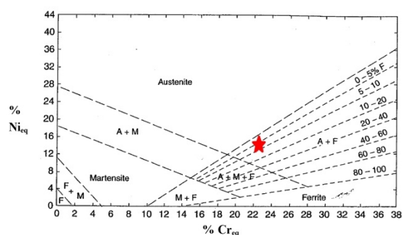
شکل 4- موقعیت کار فعلی در نمودار شفلر، که برای پیش‌بینی فازهای تشکیل‌دهنده (آستنیت ( \gamma ) و فrit دلتا ( \delta )) فولادهای زنگ‌نزن در حین انجماد با سرعت‌های سرمایش زیاد استفاده می‌شود [29].
