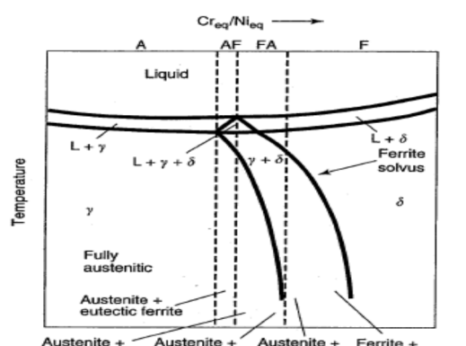
شکل 3- رابطه بین نوع انجماد و نمودار فاز شبه دوتایی [27].
