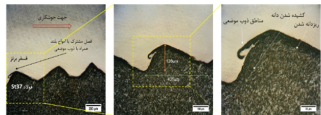
شکل 3- ریزساختار فصل مشترک اتصال نمونه شماره 1
