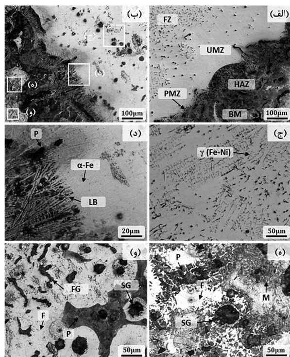
شکل 6- تصاویر میکروسکوپی نوری از نواحی مختلف چدن خاکستری جوشکاری شده به روش SMAW با الکترود ENi-CI: الف و ب- فصل مشترک FZ و BM، ج- FZ، د- UMZ و HAZ و، و- BM.
