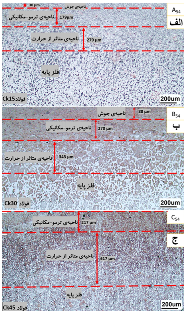
شکل 7- تصویر میکروسکوپ نوری از ریزساختار ناحیه ترمو-مکانیکی و متأثر از حرارت سه نمونه الف - A_{54} ، ب - B_{54} و ج - C_{54} در سمت ساده کربنی.
