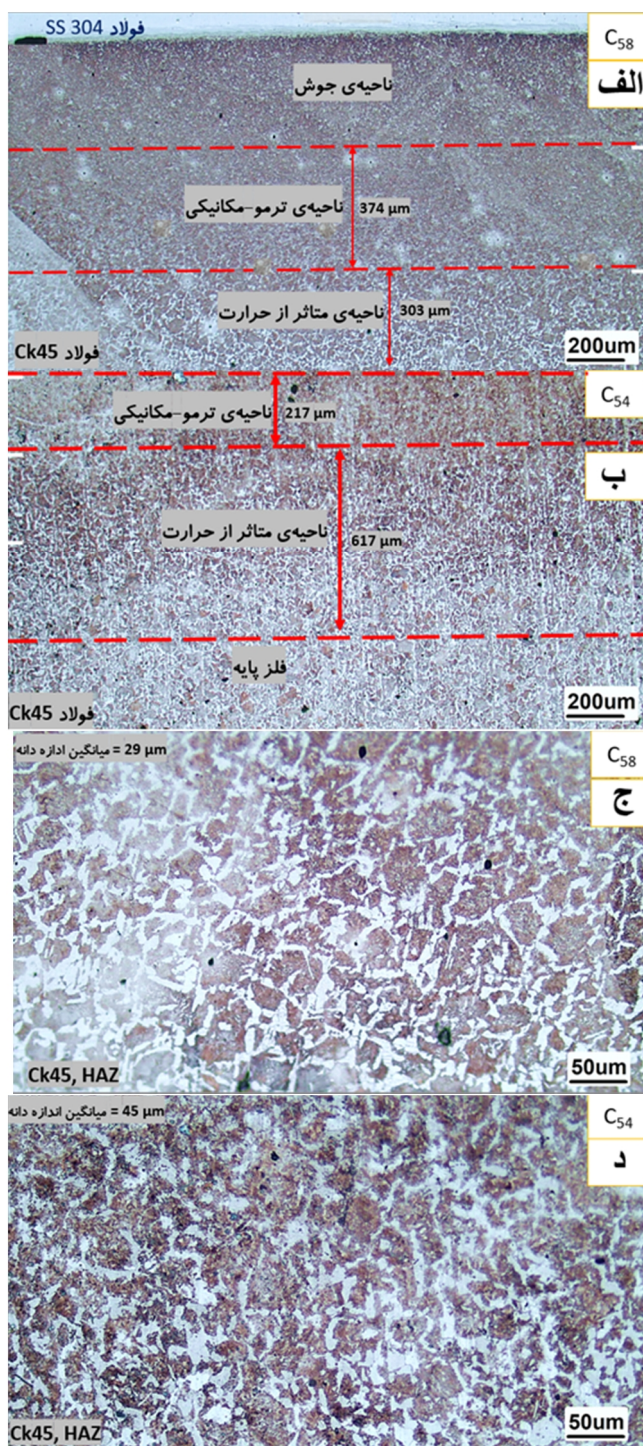
شکل 9- تصویر میکروسکوپ نوری از ریزساختار ناحیه ترمو-مکانیکی و متأثر از حرارت دو نمونه C 58 (الف و ج) و C 54 (ب و د) در سمت ساده کربنی.
