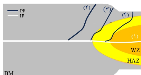
شکل 4- طرح واره مسیر انواع شکست فصل مشترکی (IF) و بیرون کشیدگی (PF) در جوشکاری مقاومتی نقطه ای.
