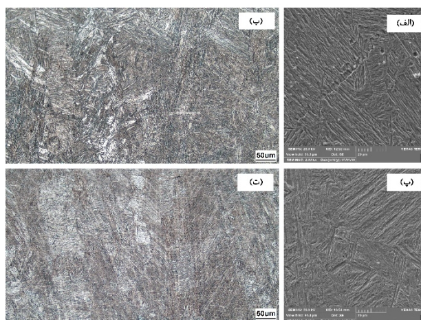
شکل 7- تصاویر میکروسکوپی الکترونی روبشی و میکروسکوپی نوری منطقه جوش در جریان 10 کیلوآمپر، الف - زمان نگهداری 5 سیکل و پ و ت - زمان نگهداری 40 سیکل.
