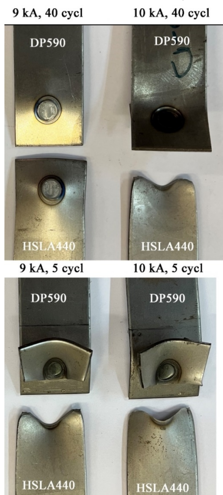
شکل 5- تصاویر شکست نمونه‌ها پس از آزمایش کشش در جریان‌های 9 و 10 و زمان‌های نگهداری 5 و 40 سیکل.
