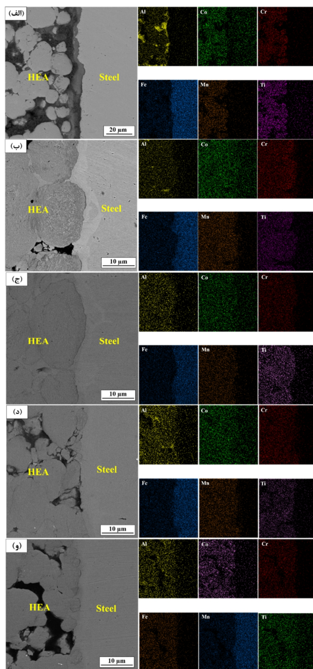
شکل 4- تصاویر FESEM و نقشه عنصری از ناحیه اتصال پوشش آلیاژ آنترپی زیاد \text{Al}_{0.5}\text{CoCrFeMnTi}_{0.5} و زیرلایه فولادی A283 در دماها و زمان های مختلف اتصال، (الف) دمای 850^{\circ}\text{C} زمان 20 دقیقه، (ب) دمای 950^{\circ}\text{C} زمان 20 دقیقه، (ج) دمای 1050^{\circ}\text{C} زمان 20 دقیقه، (د) دمای 1050^{\circ}\text{C} زمان 10 دقیقه، (و) دمای 1050^{\circ}\text{C} زمان 15 دقیقه.
