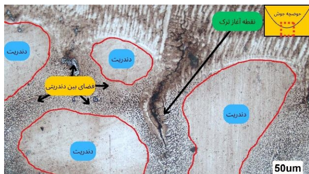
شکل 10- محل آغاز ترک در نمونه 1A-GTAW گرم بر میلی لیتر از فضای بین دندریت ها بوده است.
