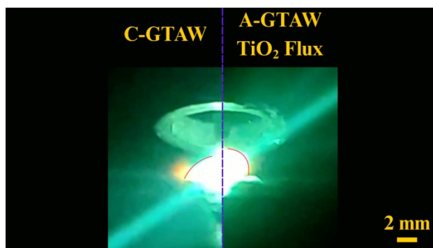
شکل 7- مقایسه عرض ناحیه متأثر از حرارت در جوشکاری بدون فلاکس و نمونه بهینه A-GTAW (1 گرم بر میلی‌لیتر).
