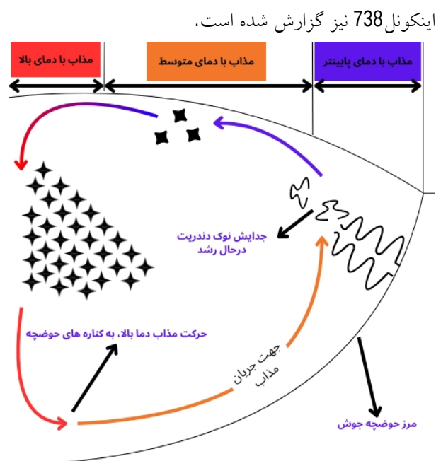
شکل 17- طرحواره از نصف سطح مقطع حوضچه که نشاندهنده اثرگذاری جریان معکوس مارانگونی بر مورفولوژی انجمادی و شکست نوک دندریت‌ها در منطقه مذاب جوشکاری قوسی تنگستن-گاز با فلاکس فعال را نشان می‌دهد.
