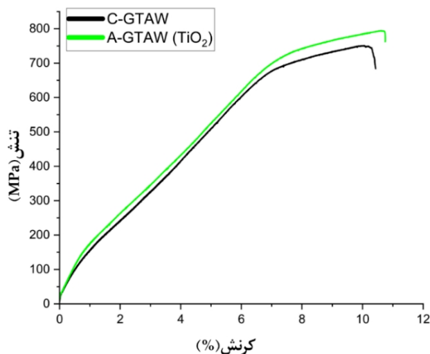
شکل 21- مقایسه رفتار تنش - کرنش نمونه‌ها با یکدیگر.
