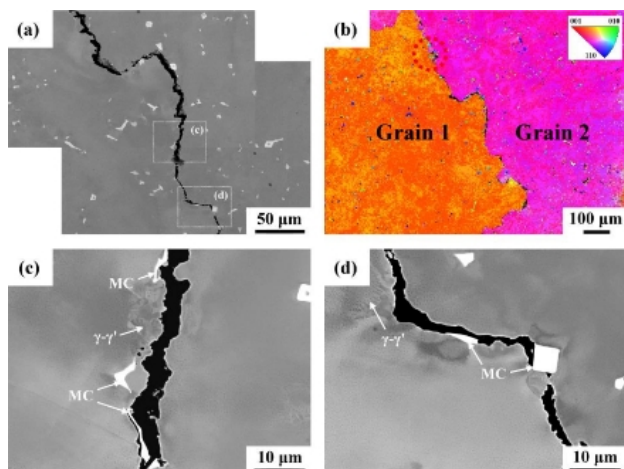
شکل 13- تصویری از ترک ذوب شدگی در منطقه HAZ، که نشان می‌دهد مسیر عبور ترک در امتداد فصل مشترک MC/ زمینه و مرزهای \gamma-\gamma' .
