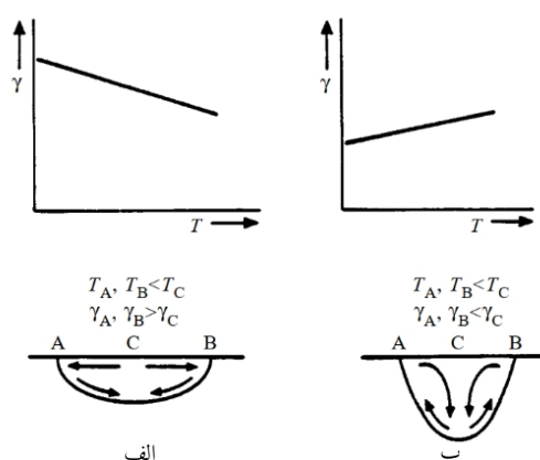
شکل 1- الف- جریان سیال در جوشکاری قوسی تنگستن-گاز مرسوم.
