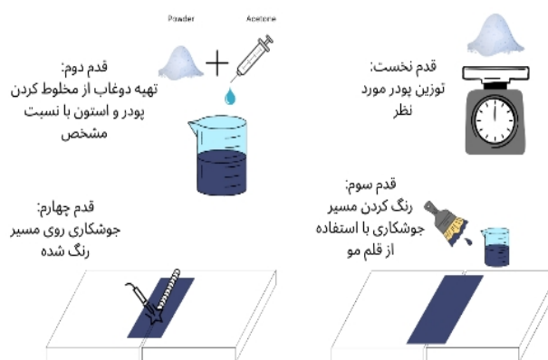
شکل 4- طرحواره ای از مراحل آماده سازی و تهیه دوغاب و نهایتاً اعمال روی سطح، پیش از جوشکاری.
