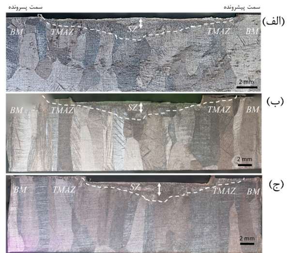
شکل 7- تصاویر درشت ساختار نمونه‌های ترمیم شده با شیارهای مختلف:
