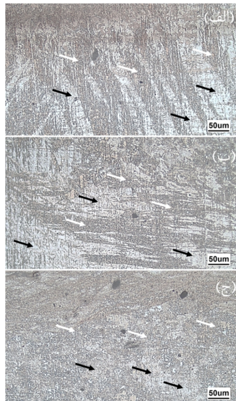
شکل 8- تصویر میکروسکوپ نوری ناحیه TMAZ در نمونه‌های ترمیم شده با شیارهای مختلف: الف- به عمق 0/5 میلی‌متر، ب- به عمق 1 میلی‌متر، ج- به عمق 1/5 میلی‌متر. نواحی تبلور مجدد یافته و نیافته به ترتیب با بیکان‌های سفید و مشکی رنگ مشخص شده‌اند.
