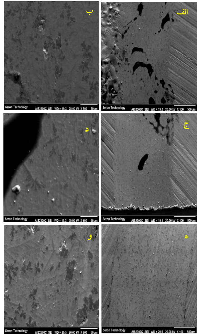
شکل 10- تصاویر شیار سایش روکش به روش قوس پلازما بعد از سایش در دمای محیط (الف و ب)، بعد از سایش در دمای 300 درجه سانتی‌گراد (ج و د) و بعد از سایش در دمای 600 درجه سانتی‌گراد (ه و و)
