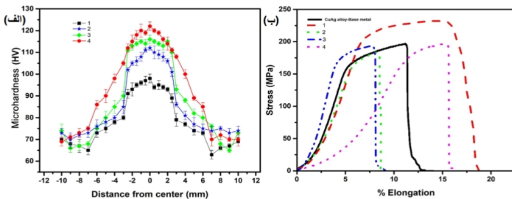
شکل 8-الف- نمودار ریزسختی سنجی ویکرز نمونه FSP شده بدون ذرات تقویت کننده (نمونه 1)، کامپوزیت Cu-Ag-SiC با ذرات تقویت کننده میکرو در مقادیر مختلف 0/02 گرم (نمونه 2) و 0/04 گرم (نمونه 3) و کامپوزیت Cu-Ag-SiC با ذرات تقویت کننده نانو (نمونه 4) و ب- منحنی‌های تنش-ازدیاد طول نمونه‌های خام، 1، 2، 3 و 4-تأثیر فرایند FSP و اندازه ذرات و مقدار تقویت کننده SiC نانومتری و میکرومتری.
