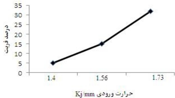
شکل 5- تغییرات فاز فریت در ریزساختار منطقه جوش براساس حرارت ورودی
