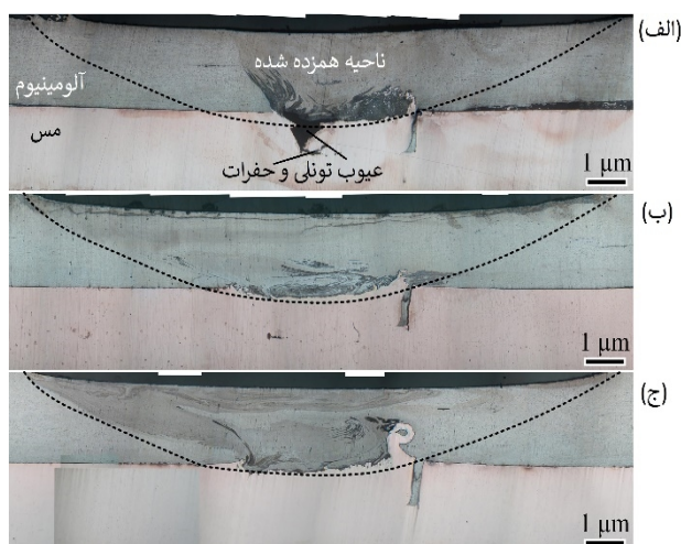
شکل 2- ماکروساختار مربوط به نمونه‌های مختلف در جهت عمود بر جهت جوشکاری همزن اصطکاکی الف - نمونه 1 (عمق نفوذ صفر)، ب - نمونه 2 (عمق نفوذ 0/05 میلیمتر) و ج - نمونه 3 (عمق نفوذ 0/1 میلیمتر).
