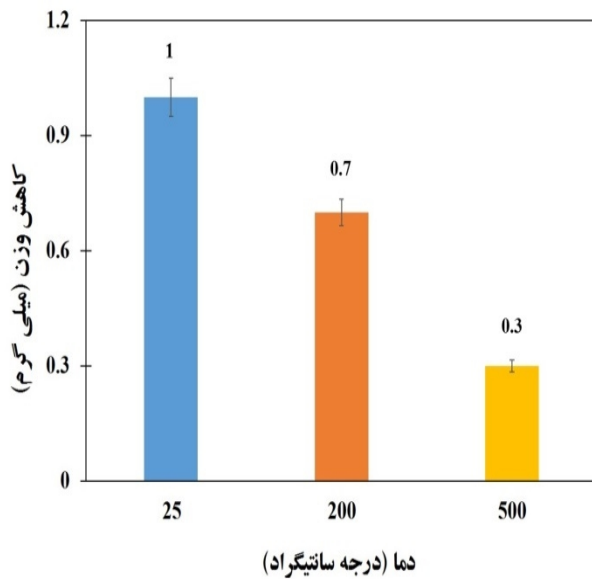
شکل 13- کاهش وزن پین‌های Fe_3Al پس از آزمایش سایش در سه دمای مختلف
