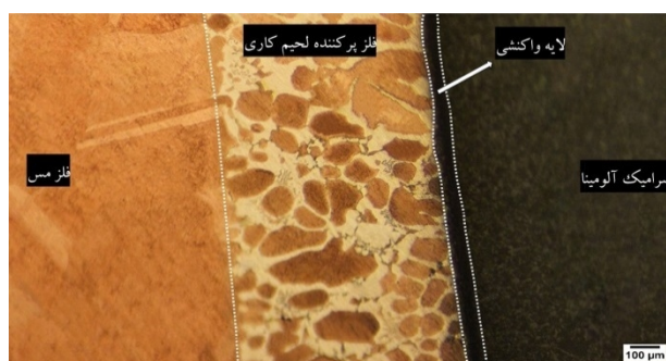
شکل 6- تصویر میکروسکوپی نوری اتصال لحیم کاری آلومینا به مس با فلز پرکننده \text{Ag-Cu-Ti-Sn-3.5Zr} .
