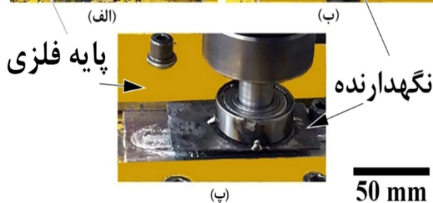
شکل 2- نحوه استفاده از پایه فلزی و نگه‌دارنده جهت جوشکاری نمونه‌ها از زوایای مختلف.
