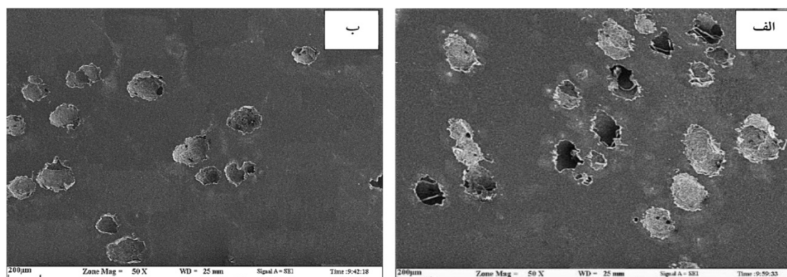
شکل 10- تصاویر SEM از مورفولوژی حفره‌های مشاهده شده در فلزجوش فولاد 17-4PH در شرایط: الف- as-weld و ب- فرایپرسازی دومرحله.
