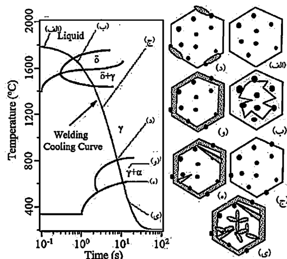
شکل 4- نمودار منحنی سرمایش و تشکیل فازهای مختلف در دکه جوش [22].
