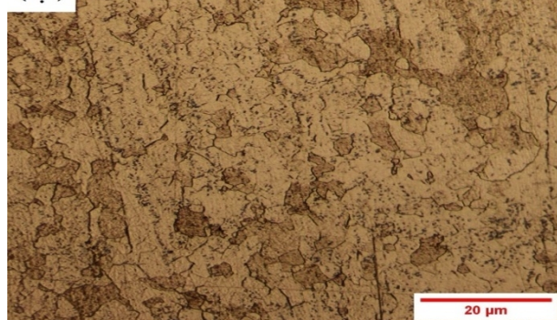
شکل 2- الف - ریزساختار فولاد S500 MC در بزرگنمایی 500 برابر و ب - ریزساختار AISI 430 در بزرگنمایی 100 برابر (مقطع RD-TD).
