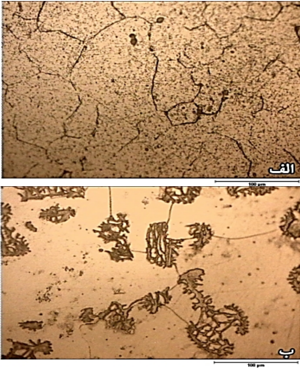
شکل 1- ریزساختار فلزات پایه (الف) سوپراآلیاژ (در دمای °C 1170 به مدت 30 دقیقه آنیل و در آب کوئنچ شده) (ب) ترکیب بین فلزی Ni 3 Al.
