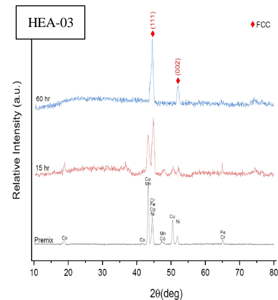
شکل 4- آنالیز XRD سه ترکیب پودر پرکننده.
