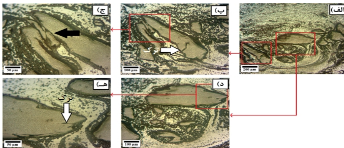
شکل 7- تصویر میکروسکوپی نوری ریزساختار منطقه کامپوزیتی نمونه جوشکاری شده با سرعت چرخش 250 دور در دقیقه و سرعت پیشروی 20 میلی متر بر دقیقه الف - قسمتی از منطقه اغتشاشی، ب-ه- تصاویر متناظر با بزرگنمایی بالاتر.
