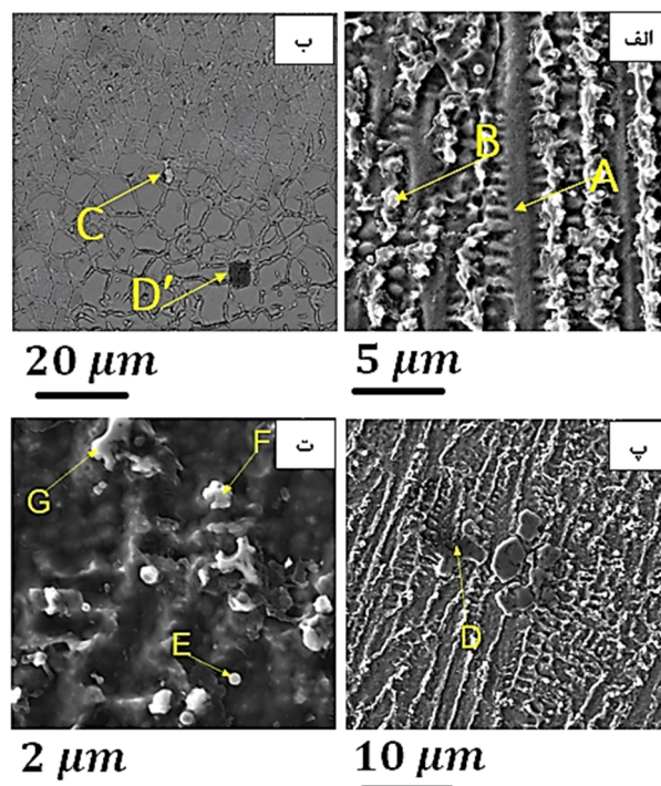
شکل 8- آنالیز عنصری از نقاط تعیین شده در بزرگ‌نمایی‌های مختلف.
