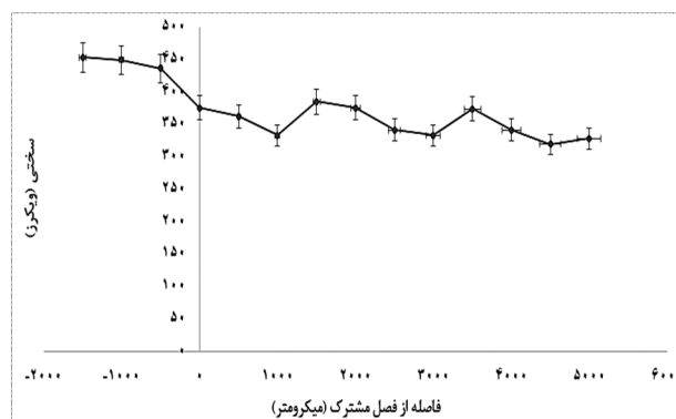
شکل 10- پروفیل سختی پره IN713LC تعمیر شده توسط اینکونل 625.
