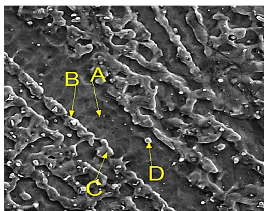
شکل 9- تصویر میکروسکوپی الکترونی روبشی از سطح و نقاط مشخص شده جهت آنالیز.
