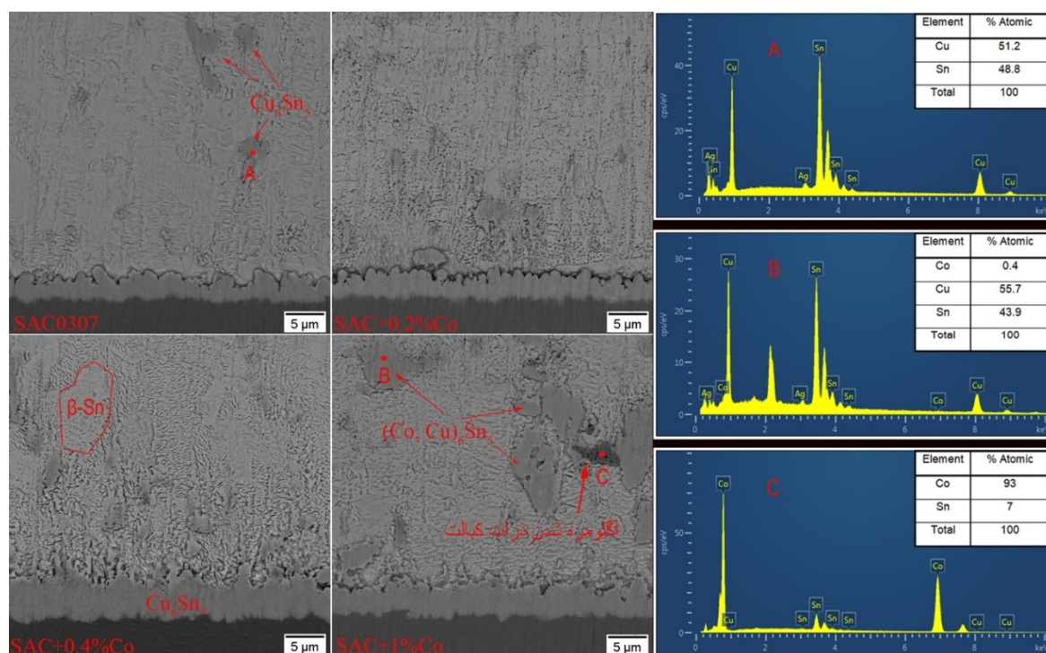
شکل 8- تصاویر ریزساختاری فصل مشترک لحیم‌های کامپوزیتی حاوی درصدهای مختلف ذرات کبات.
