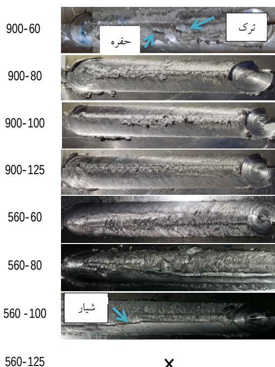
شکل 6- کیفیت ظاهری نمونه ها در شرایط سرعت چرخشی 560 و 900 rpm و سرعت های پیشروی مختلف.
