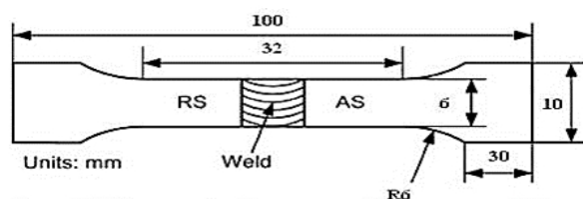
شکل 5- شکل و ابعاد نمونه‌های آزمون کشش
