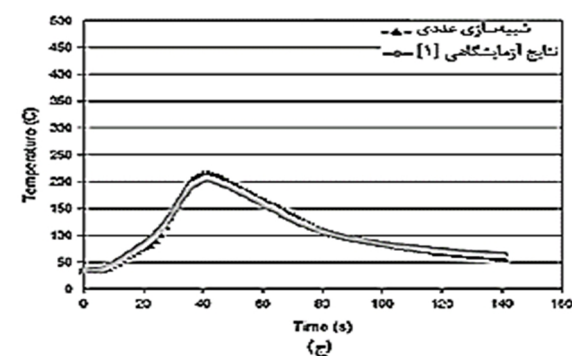
شکل 4- نتایج شبیه‌سازی عددی و نتایج آزمایشگاهی در قطعه کار و مقایسه آن با دمای پیش‌بینی شده در سرعت دورانی 350 دور بر دقیقه و سرعت پیشروی ابزار 3 میلی‌متر بر ثانیه و در سه فاصله مختلف، الف- 7 میلی‌متر، ب- 15 میلی‌متر، ج- 25 میلی‌متر از خط جوش.
