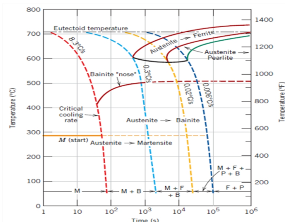
شکل 7- دیاگرام TTT فولاد 4340- [18]
