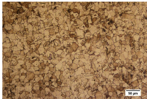
شکل 1- ریزساختار فولاد AISI 316L.
