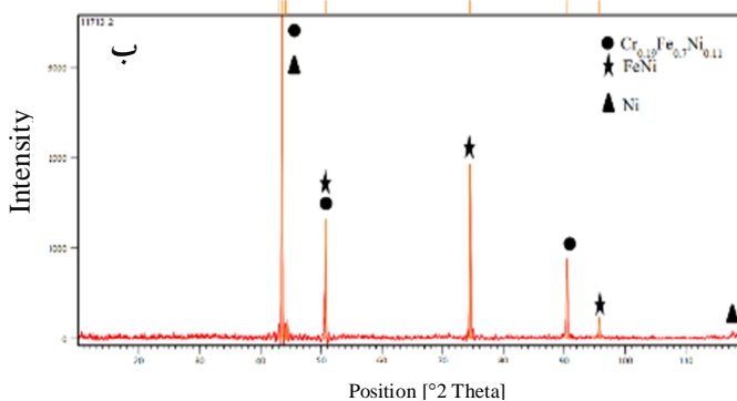
شکل 5- بررسی XRD موضع اتصال. الف- قبل از تکمیل انجماد هم‌دما ( 1050^{\circ}\text{C}/5\text{ min} )، ب- بعد از تکمیل انجماد هم‌دما ( 1050^{\circ}\text{C}/20\text{ min} ).
