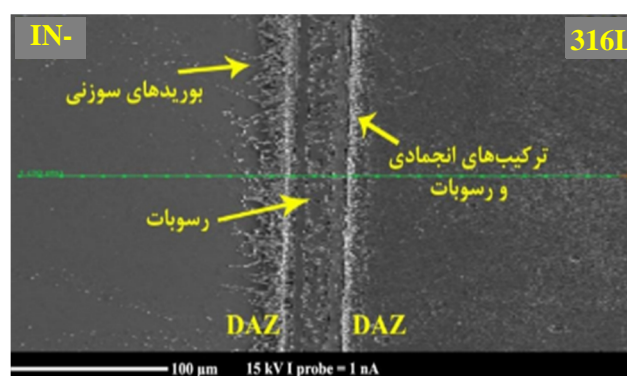
شکل 7- تصویر میکروسکوپ الکترونی از ترکیبات ناحیه DAZ
