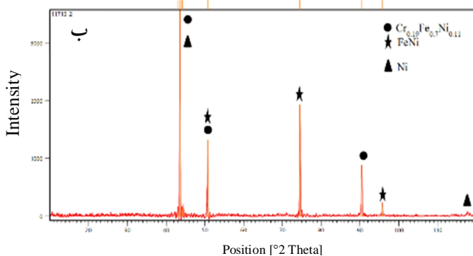
شکل 5- بررسی XRD موضع اتصال. الف- قبل از تکمیل انجماد همدا (1050 °C/20 min)، ب- بعد از تکمیل انجماد همدا (1050 °C/20 min).
