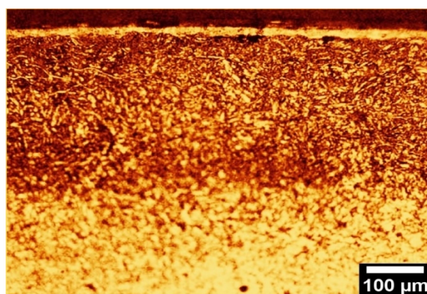
شکل 3- تصویر میکروسکوپ نوری از ریزساختار فلز پایه DIN 34CrAlNi7 نیتروژن دهی شده
