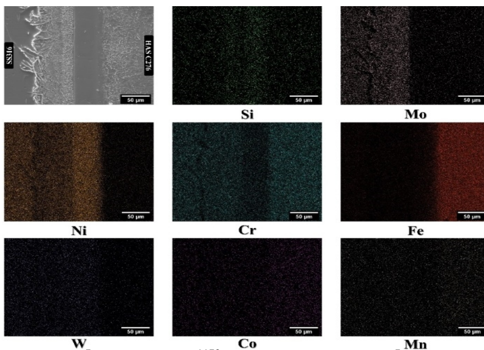
شکل 5- نقشه EDS اتصالات انجام شده در دمای 1150 درجه سانتی‌گراد و زمان 5 دقیقه
