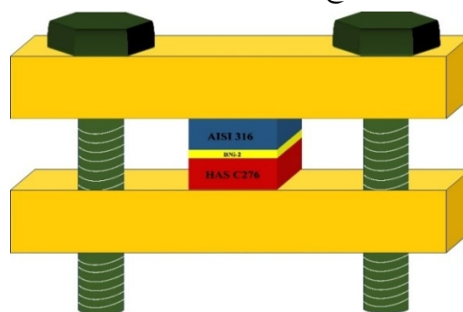
شکل 1- شماتیک نگه دارنده فرایند اتصال فاز مایع گذرا
