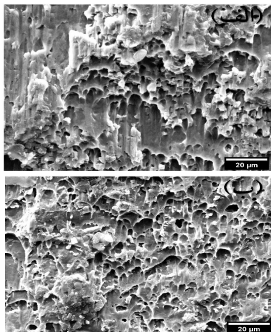
شکل 10- تصویر میکروسکوپ الکترونی روبشی از سطح شکست اتصال انجام شده در دمای 1150 درجه سانتی‌گراد الف - 5 دقیقه و ب - 30 دقیقه
