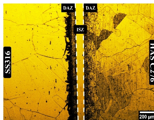
شکل 3- تصویر میکروسکوپ نوری (OM) اتصال انجام‌شده در دمای 1150 درجه سانتی‌گراد و زمان 5 دقیقه
