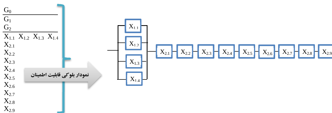
شکل 2- مجموعه‌های برشی و نمودار بلوکی قابلیت اطمینان سیستم.
