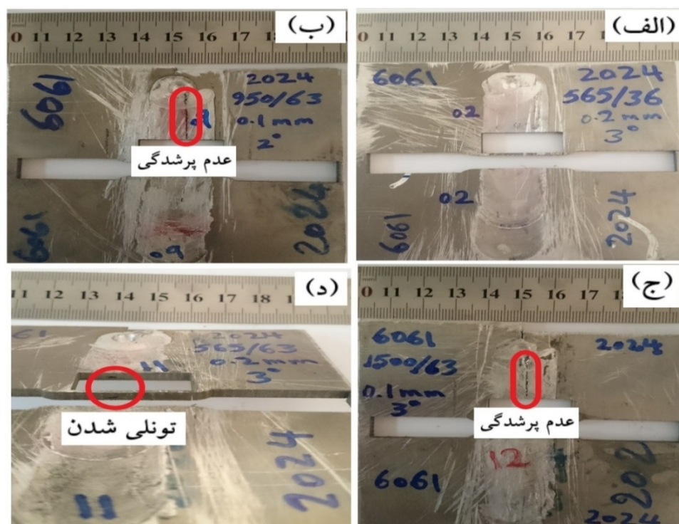
شکل 2- الف- نمونه 2 جوش بدون عیب ب- عیب عدم پرشدگی در نمونه 9 ج- عیب عدم پرشدگی در نمونه 12 و د- عیب عدم پرشدگی و تونی شدن در نمونه 11
