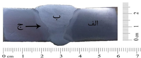
شکل 2- مقطع نمونه جوشکاری شده فولاد P460NH با الکتروکود E8018-G الف- فلز پایه ب- ناحیه جوش ج- ناحیه متأثر از حرارت (حکاکی شده توسط محلول‌های پیکرال 2 درصد و نایتال 2 درصد).
