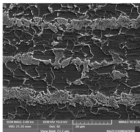
شکل 4- میکروسکوپ الکترونی روبشی از ریز ساختار فلز پایه از فلز پایه (حکاکای شده توسط محلول‌های پیکرال 2 درصد و نایتال 2 درصد).
