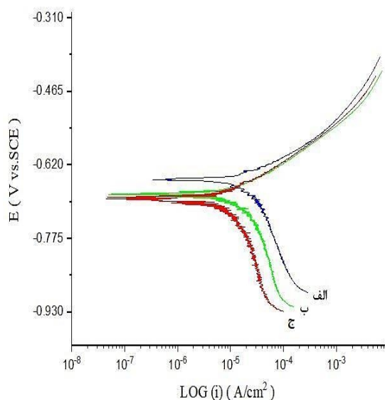
شکل 12- منحنی پلاریزاسیون تافل (الف) ناحیه متأثر از حرارت، (ب) فلز جوش، (ج) فلز پایه.
