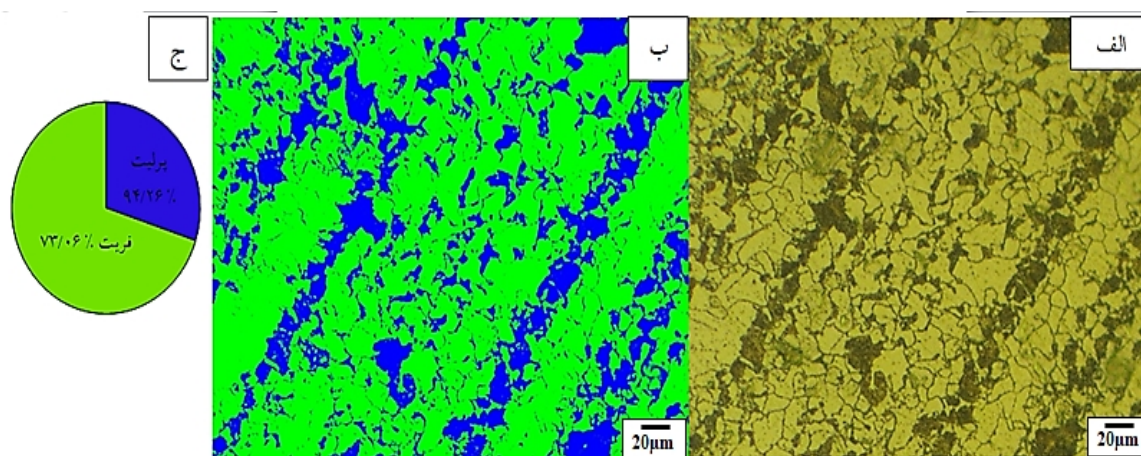
شکل 3- الف- تصویر میکروسکوپ نوری از ریزساختار فلز پایه (حکاکای شده توسط محلول‌های پیکرال 2 درصد و نایتال 2 درصد) ب- آنالیز فازی تصویری ج- درصد فازی.
