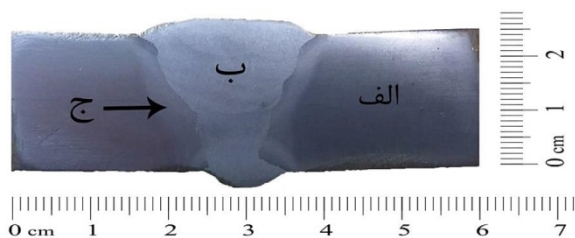
شکل 2- مقطع نمونه جوشکاری شده فولاد P460NH با الکتروود E8018-G الف - فلز پایه ب - ناحیه جوش ج - ناحیه متأثر از حرارت (حکاکی شده توسط محلول‌های پیکرال 2 درصد و نایتال 2 درصد).
