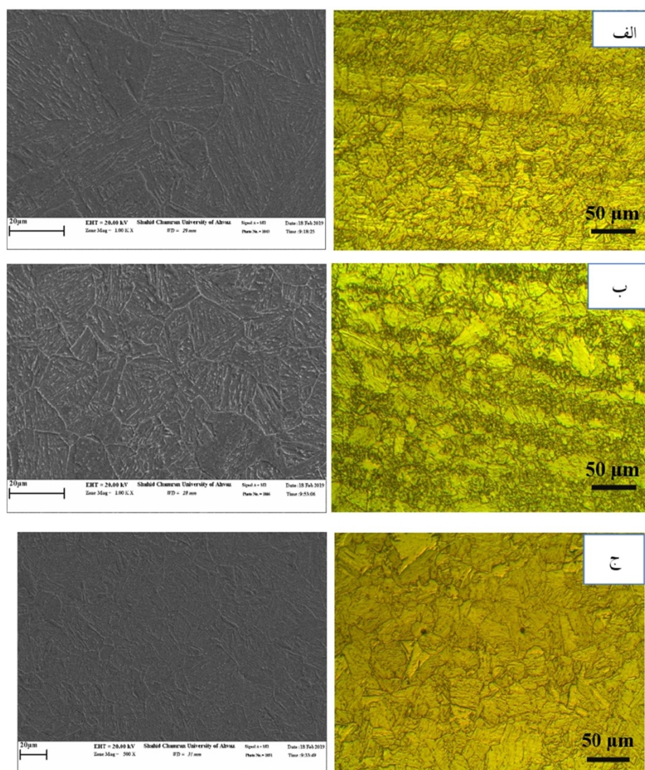
شکل 3- تصاویر میکروسکوپ نوری و الکترونی روبشی از ریزساختار ناحیه CGHAZ در حرارت‌های ورودی مختلف الف- 0/82 ب- 1/176 ج- 1/392 کیلوژول بر میلی‌متر.
