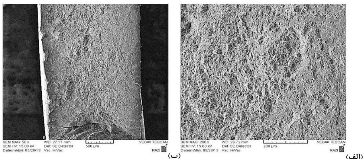
شکل 11- ماکروگراف SEM نمونه کشش عرضی آلایژ ریختگی 7075 قرآوری شده اغتشاشی اصطکاکی، (الف) حضور لبه های برشی، (ب) حضور تورفتگی های نسبتا کوچک.
