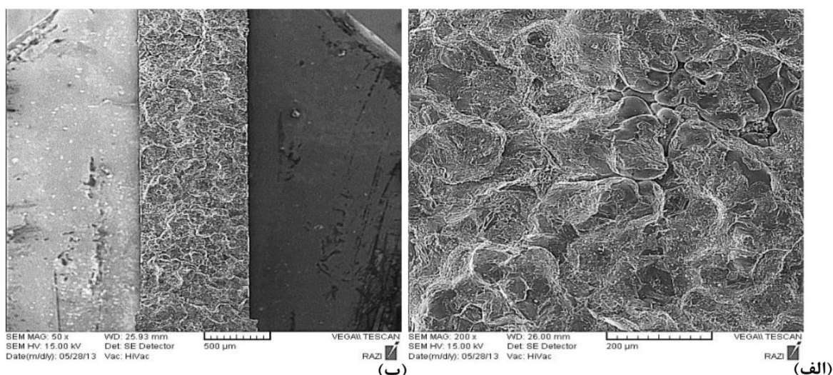
شکل 10- ماکروگراف های SEM سطح شکست آزمایش کشش عرضی نمونه ریختگی آلایژ آلومینیوم 7075، (الف) عدم حضور لبه های برشی و (ب) حضور چاک های تیره (حفرات انقباضی).
