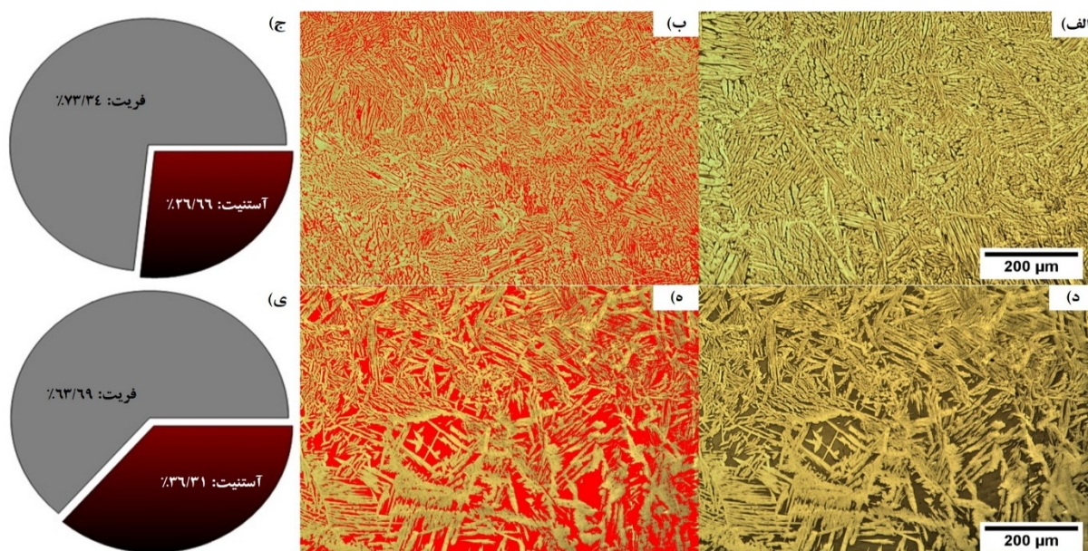
شکل 1- ریزساختار فلز جوش ER2209، (الف) پاس ریشه، (ب) آنالیز فازی تصویری پاس ریشه، (ج) آنالیز فازی عددی پاس ریشه، (د) پاس آخر، (ه) آنالیز فازی تصویری پاس آخر و (و) آنالیز فازی عددی پاس آخر
