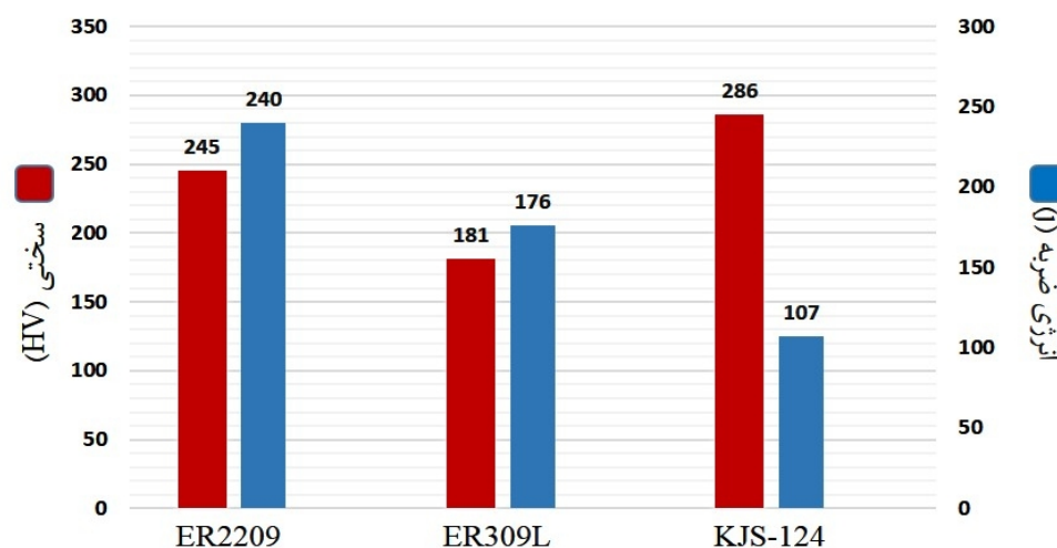
شکل 8- نتایج آزمون ضربه و سختی
