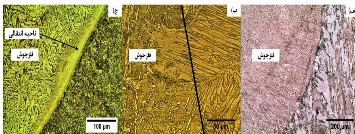
شکل 4- فصل مشترک فلز جوش ER2209 با فلزهای پایه (الف) DSS 2205، (ب) DSS 2205 با بزرگنمایی بیشتر و (ج) API 5L X80
