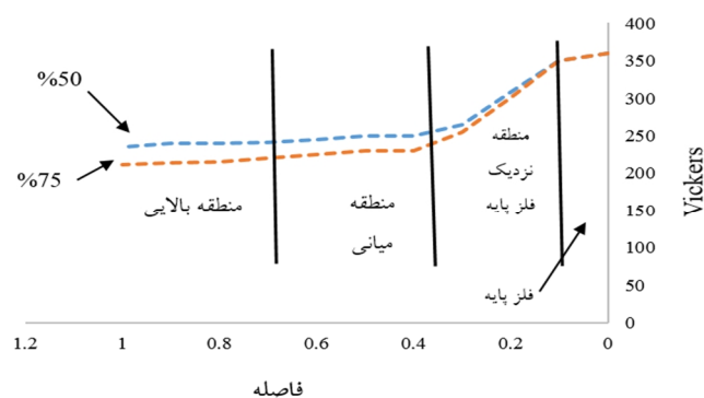
شکل 7- نمودار ریزسختی پوشش با هم پوشانی تک پاس های روکش 50 و 75 درصد
