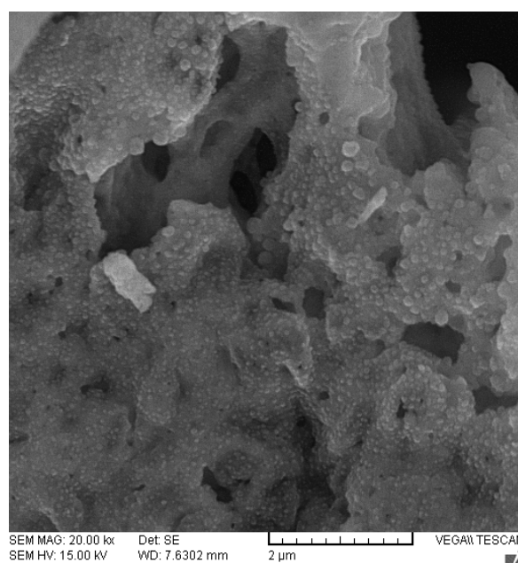
شکل 11 - تصویر میکروسکوپی الکترونی نمونه شماره 1.
