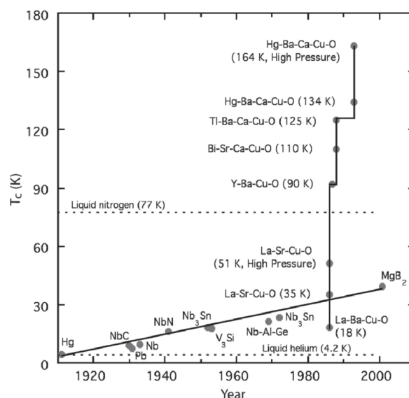
شکل 1- دمای بحرانی مواد ابرسانی دما پایین و بالا [7].
