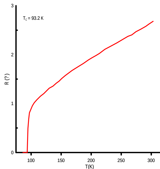
شکل 20 - نمودار آزمون رسانایی چهارنقطه‌ای فیلم نازک ابرسانا.
