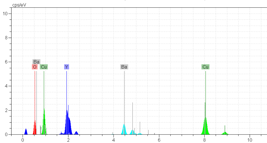
شکل 18- الگوی پراش انرژی اشعه ایکس نمونه شماره 3.
