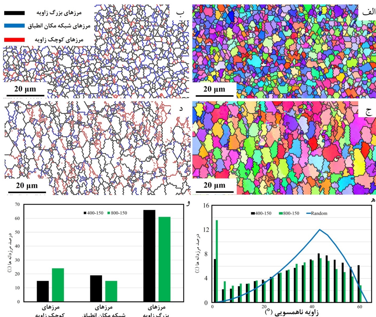
شکل 3- الف) و ب) نقشه جهت‌گیری و مرزدانه‌ای SZ نمونه 400 دور بر دقیقه، ج) و د) نقشه جهت‌گیری و مرزدانه‌ای SZ نمونه 800 دور بر دقیقه، ه) و و) منحنی توزیع زوایای ناهمسوئی و منحنی درصد نوع مرزدانه‌ها.
