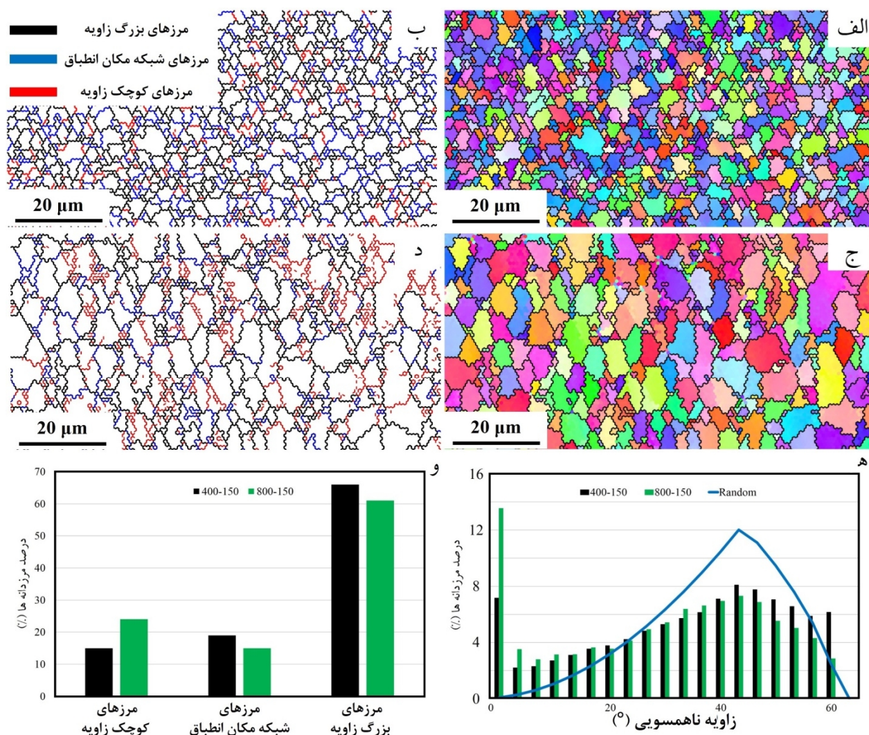
شکل 3- الف) و ب) نقشه جهت‌گیری و مرزخانه‌های SZ نمونه 400 دور بر دقیقه، ج) و د) نقشه جهت‌گیری و مرزخانه‌های SZ نمونه 800 دور بر دقیقه، ه) و و) منحنی توزیع زوایای ناهمسویی و منحنی درصد نوع مرزخانه‌ها.
