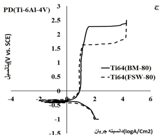
شکل 9- منحنی‌های پتانسیودینامیک Ti-6Al-4V در شرایط جوهرکاری اصطکاکی همزنی در محلول 3/5 NaCl در دماهای الف) 25، ب) 37، ج) 80 درجه سانتی گراد.
