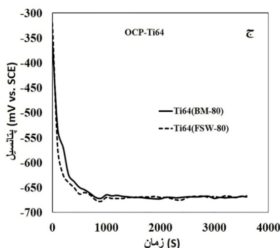
شکل 8- تغییرات پتانسیل مدار باز آلیاژ \text{Ti-6Al-4V} در 3/5 درصد \text{NaCl} (الف) 25، (ب) 37، (ج) 80 درجه سانتی گراد.
