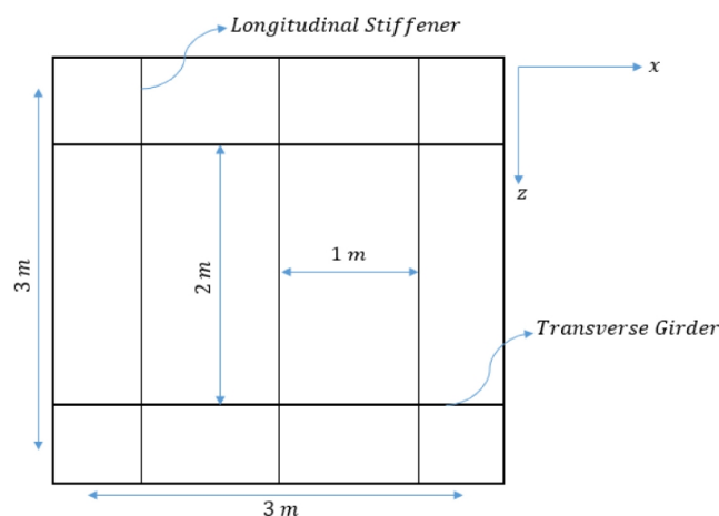
شکل 11- سیستم فریم‌بندی طولی در پانل بزرگ
