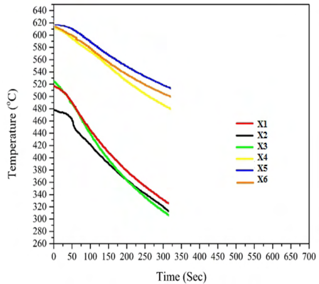
شکل ۹- نمودار سرد شدن نمونه های جوش
