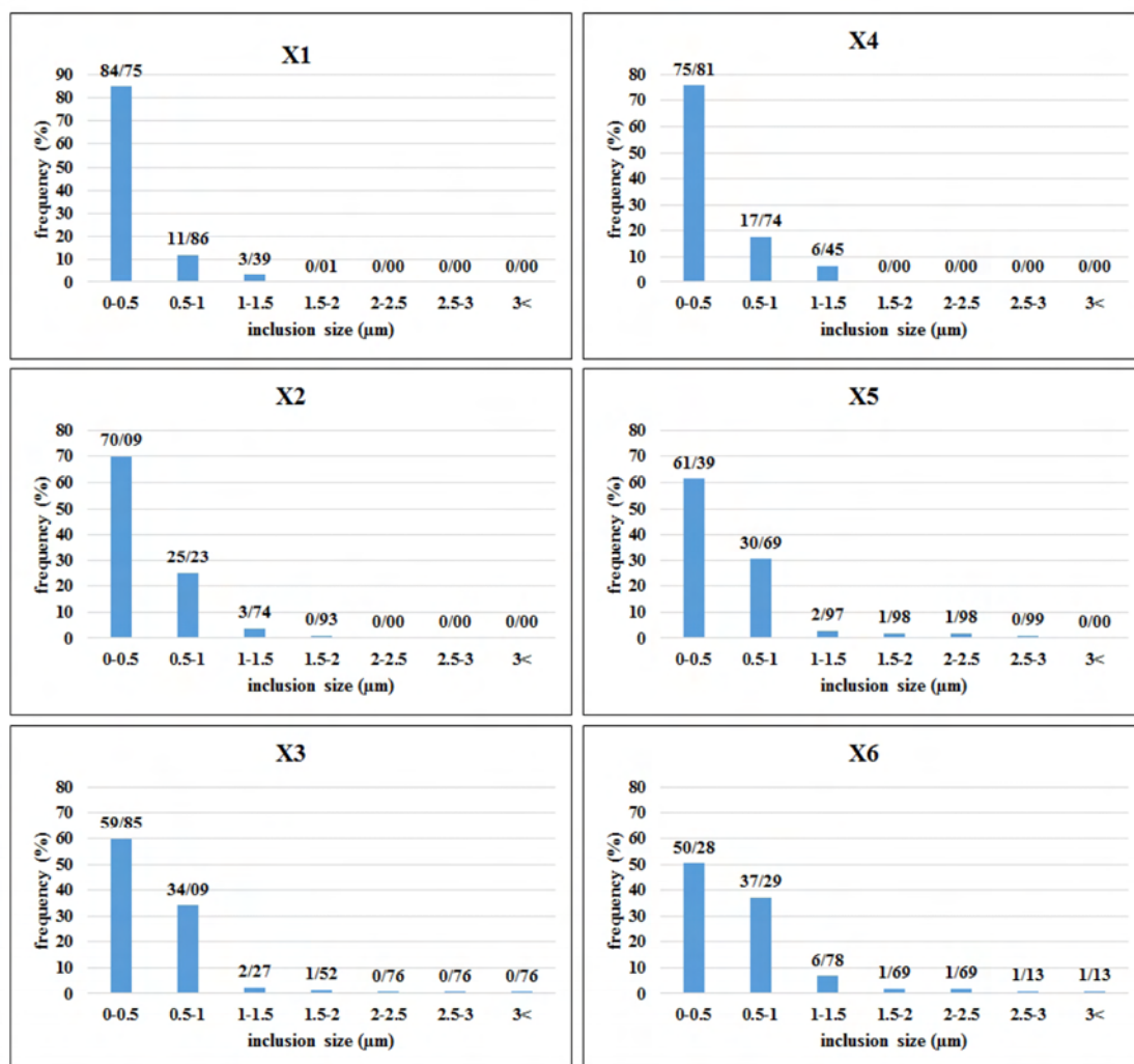
شکل 4- توزیع اندازه آخالهای تشکیل یافته در نمونه های جوش
