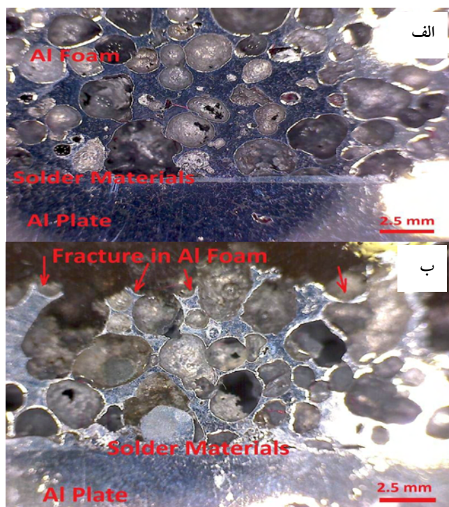
شکل ۴-الف) محل اتصال فوم آلومینیوم به همراه ورق پیش از آزمون کشش، ب) فصل مشترک مورد آزمون و شکست فوم .
