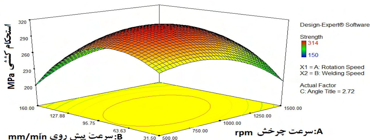
شکل 9- اثر پارامترهای متغیر سرعت دورانی و سرعت خطی ابزار بر روی استحکام کششی ورق های جوش خورده.
